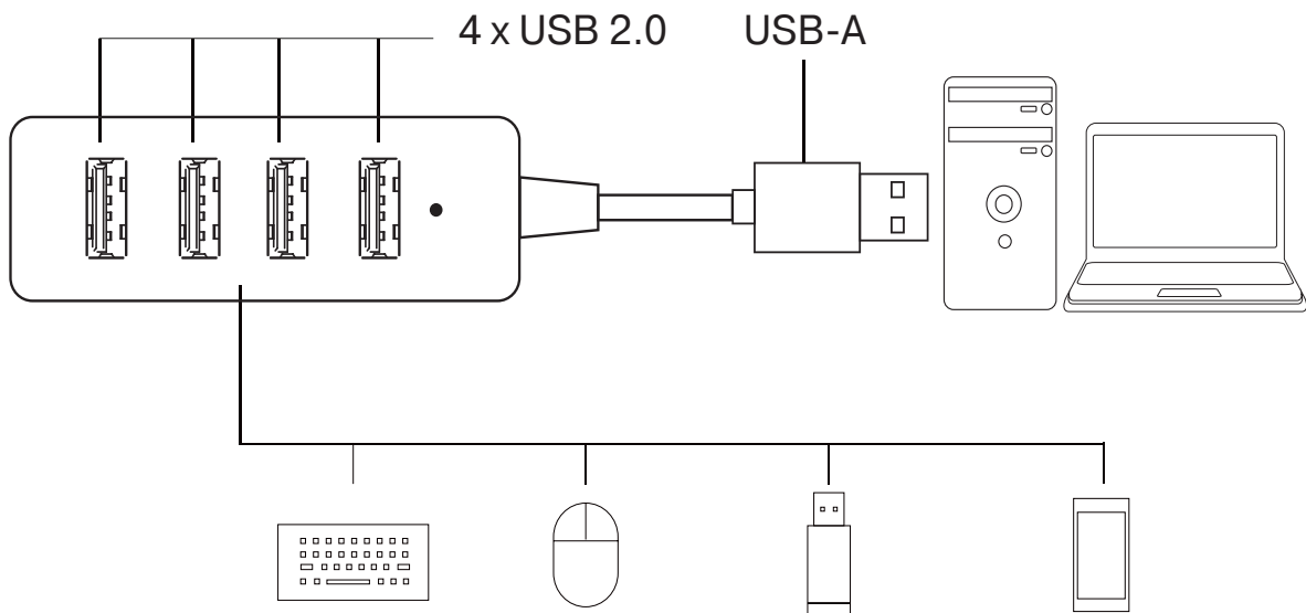
Схема подключения
